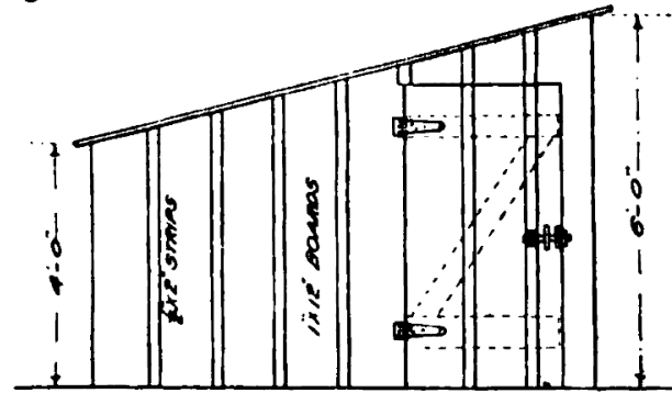
END ELEVATION
